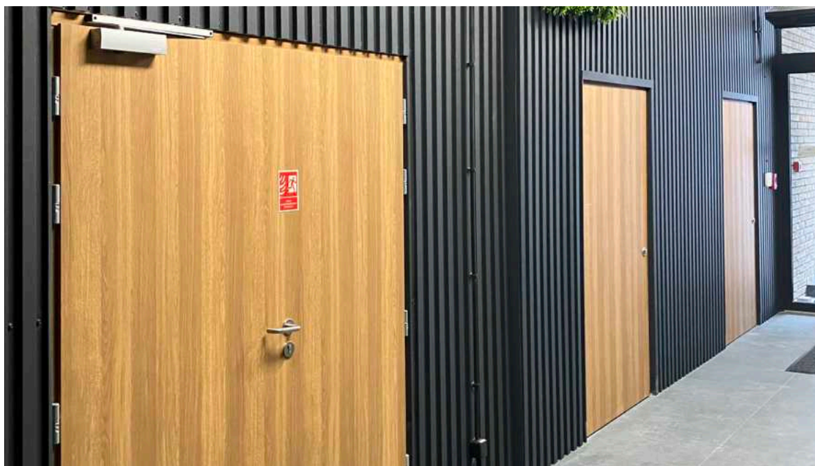
dvoukřídlé dveře EI30 PLUS, nastavitelná dřevěná zárubeň
