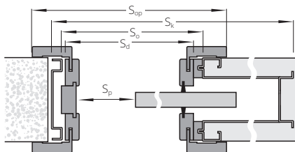
SYSTÉM POSUVNÝ: DVEŘE DO STAVEBNÍHO POUZDRA:
