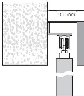
nástěnný posuvný systém s tunelovou zárubní ZN (neplatí pro systém PREMIUM)
