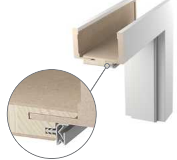
SOLID DIN DUO vyrobena z vysoce kvalitního vrstveného dřeva (základní část), lišty vyrobeny z vysoce kvalitní MDF
